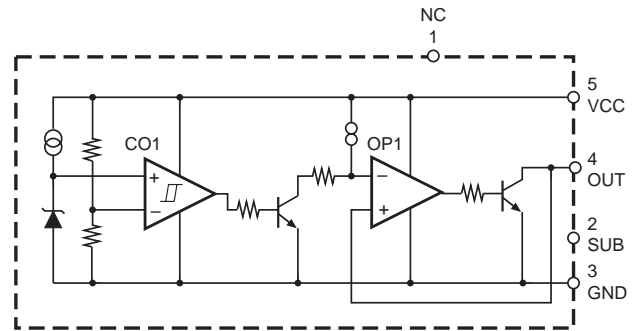
Fig. 6.4 Voltage Detector PST9142NR (U303)
